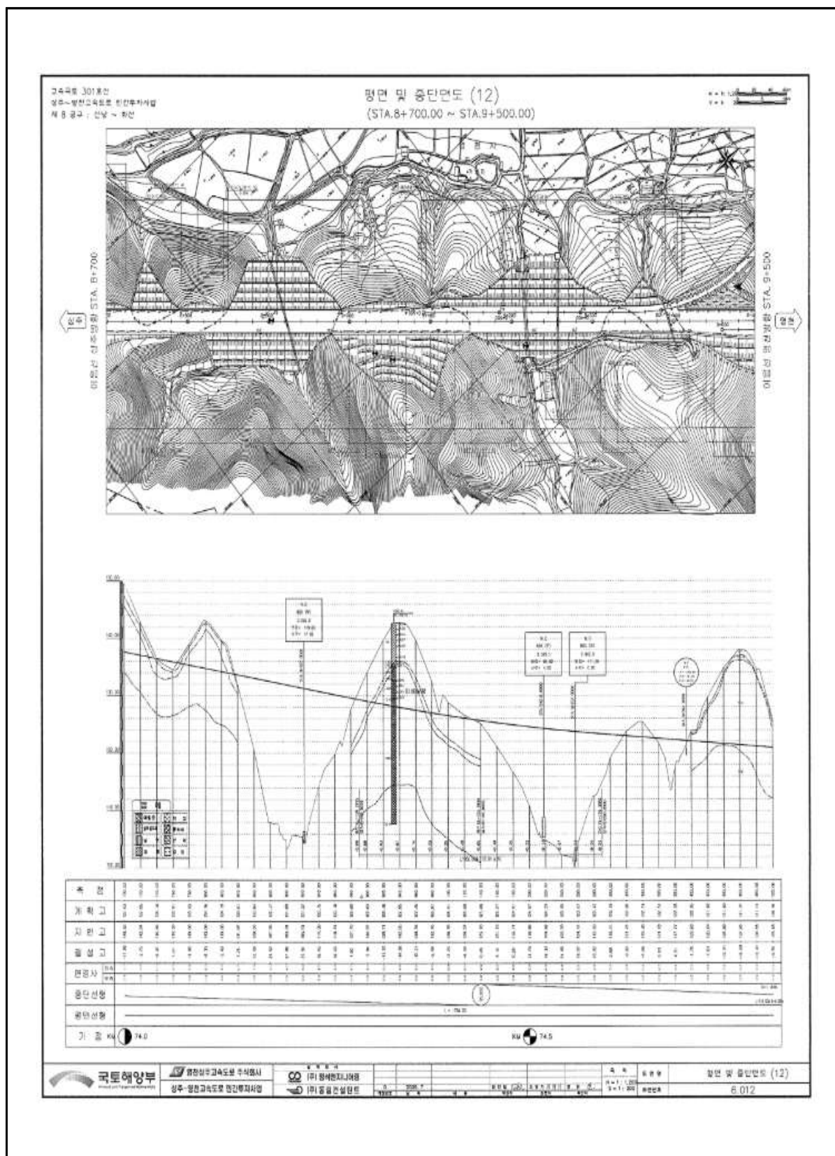
【표 55-3】 평면도
