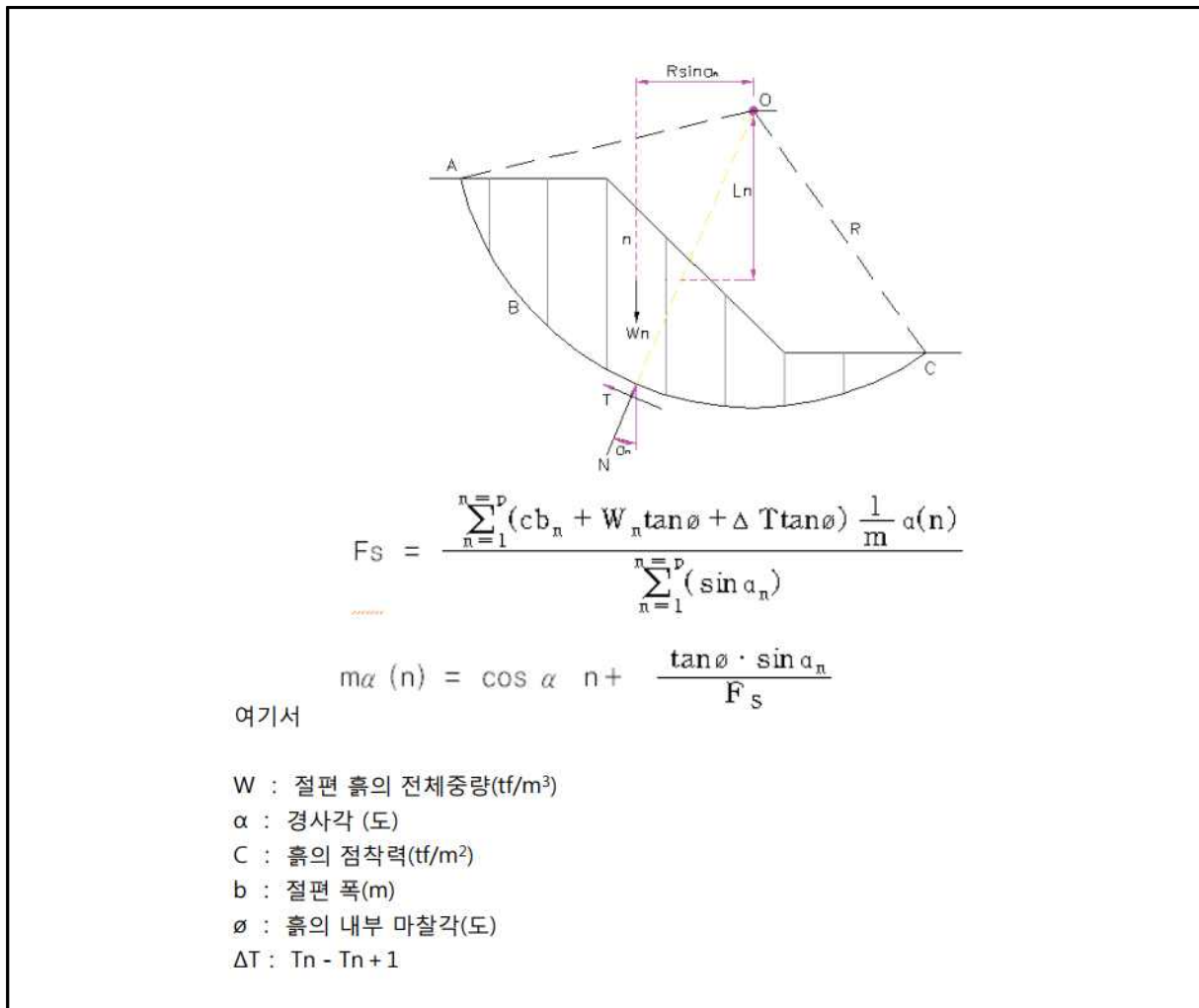
【표 55-50】 Bishop의 안전율 계산식
